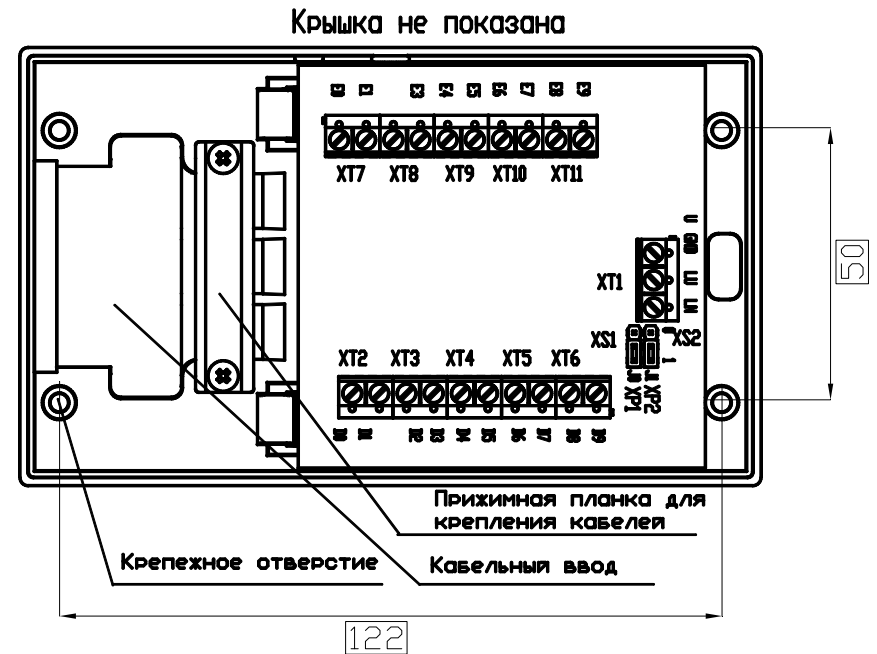
Рис. 2. Внешний вид КМ100-7.3
