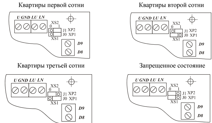
Рис.3 Положение джамперов XP1, XP2 и XP3 для различного диапазона квартир
